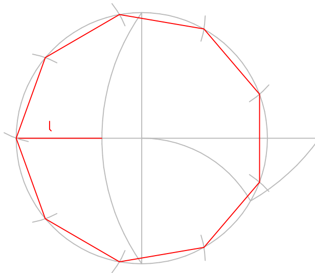
División circunferencia en 9 partes
