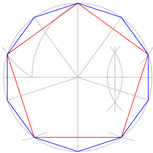
División circunferencia en 5 - 10 partes
