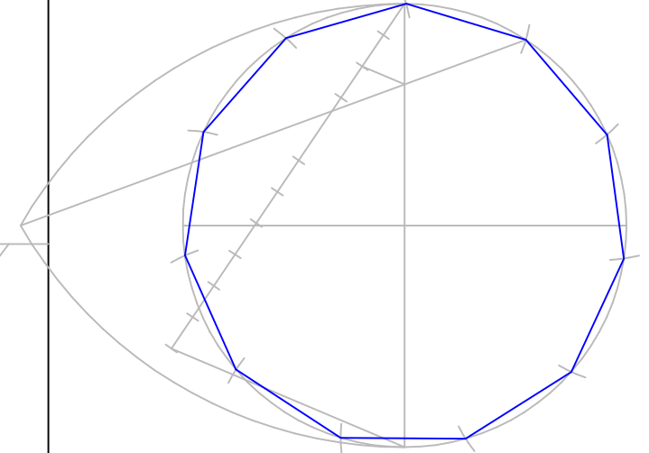
División circunferencia en N partes (11)
