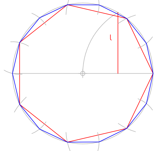
División circunferencia en 7 - 14 partes
